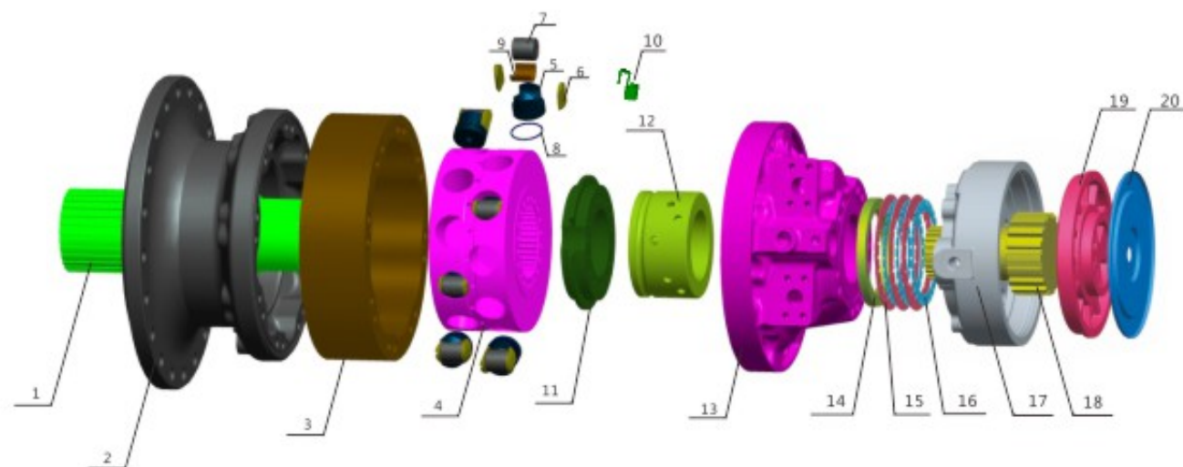
HMS83 系列零件名称表 HMS83 series parts list
