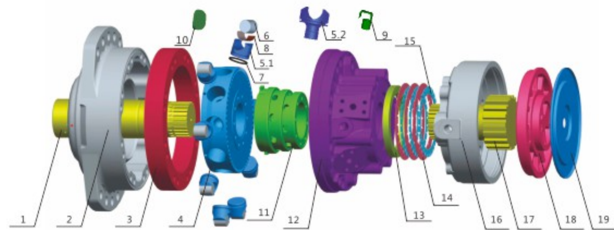
HMS18/HMSE18 系列零件名称表 HMS18/HMSE18 series parts list
