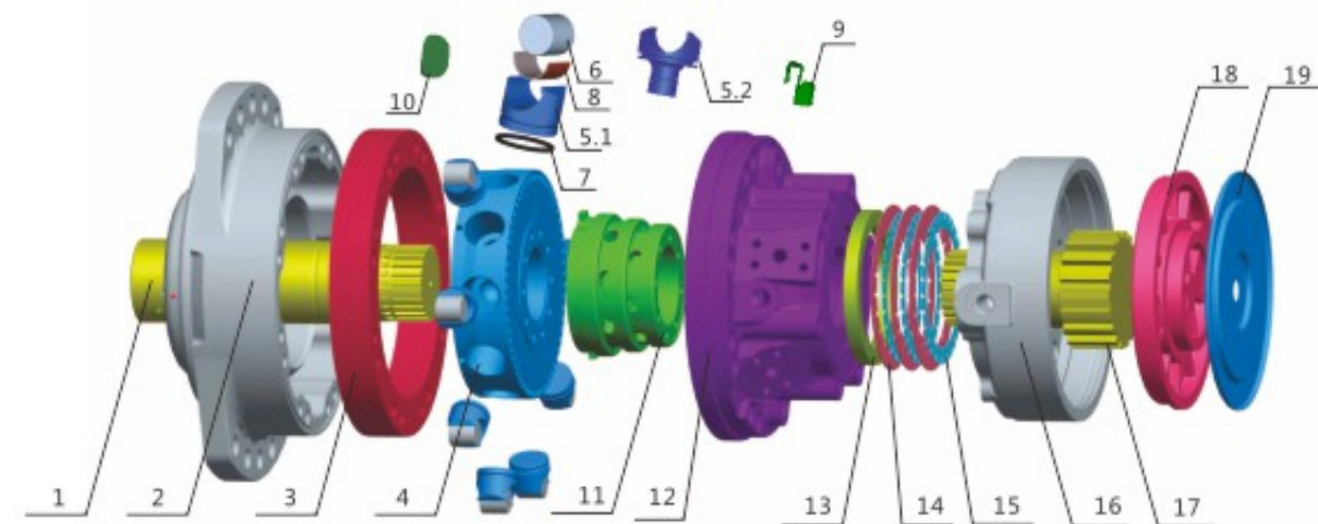
HMS08/HMSE08 系列零件名称表 HMS08/HMSE08 series parts list
