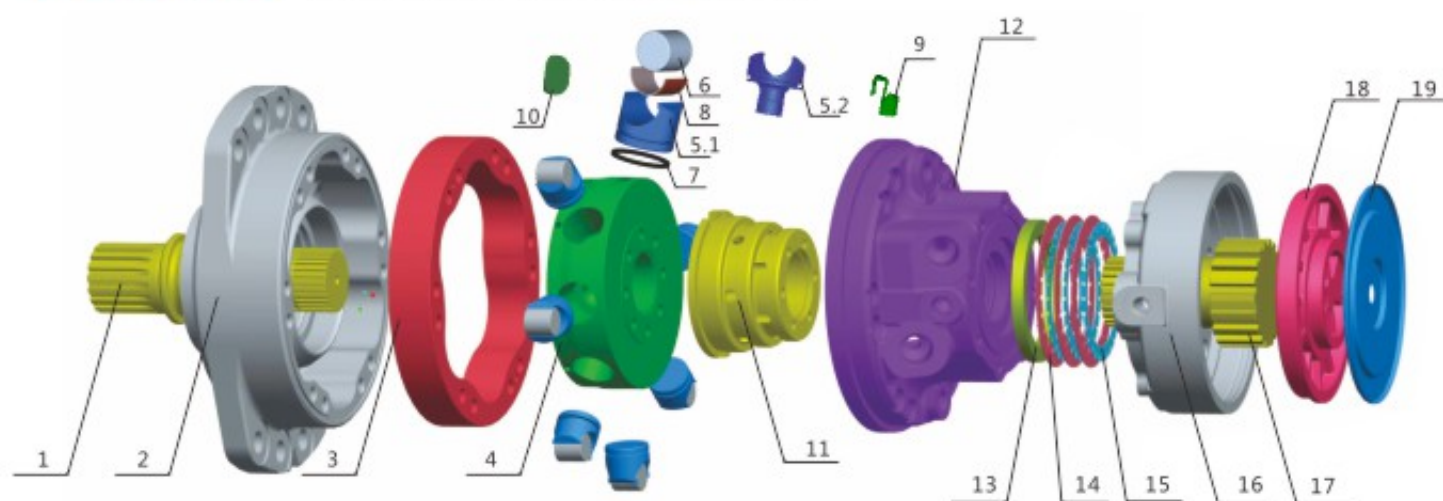
HMS05/HMSE05 系列零件名称表 HMS05/HMSE05 series parts list
