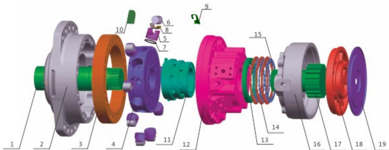
HMS25 系列零件名称表 HMS25 series parts list
