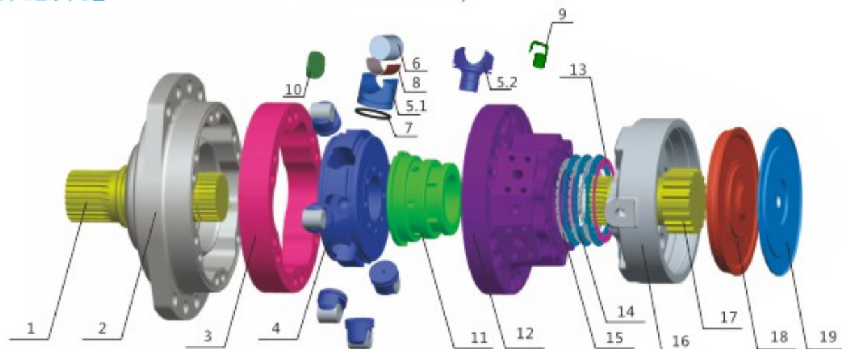
HMS11/HMSE11 系列零件名称表 HMS11/HMSE11 series parts list
