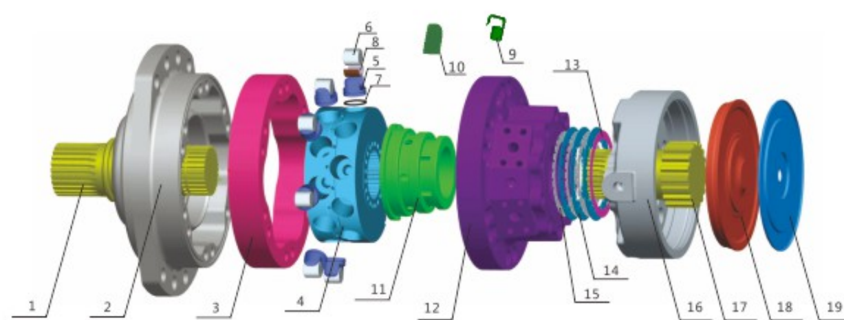
HMS35 系列零件名称表 HMS35 series parts list
