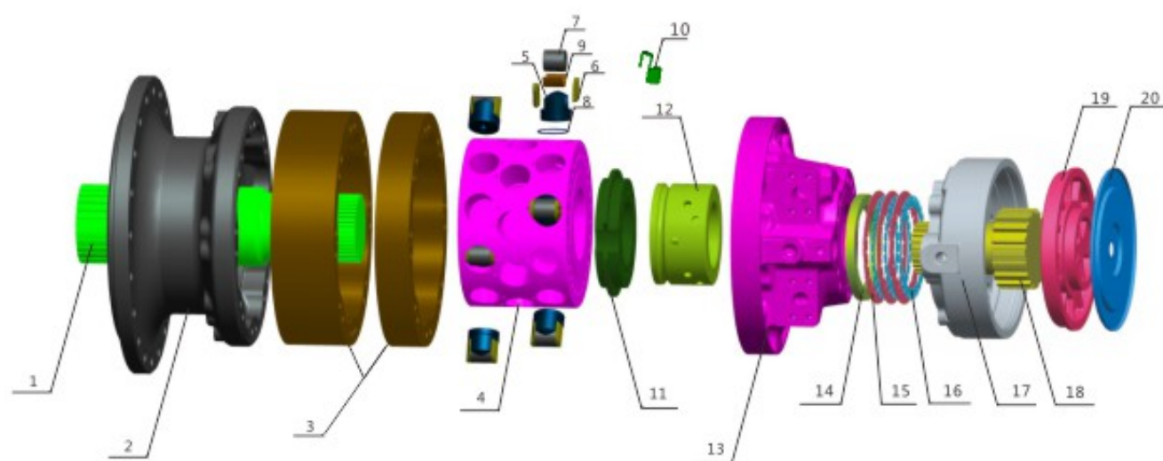
HMS125 系列零件名称表 HMS125 series parts list
