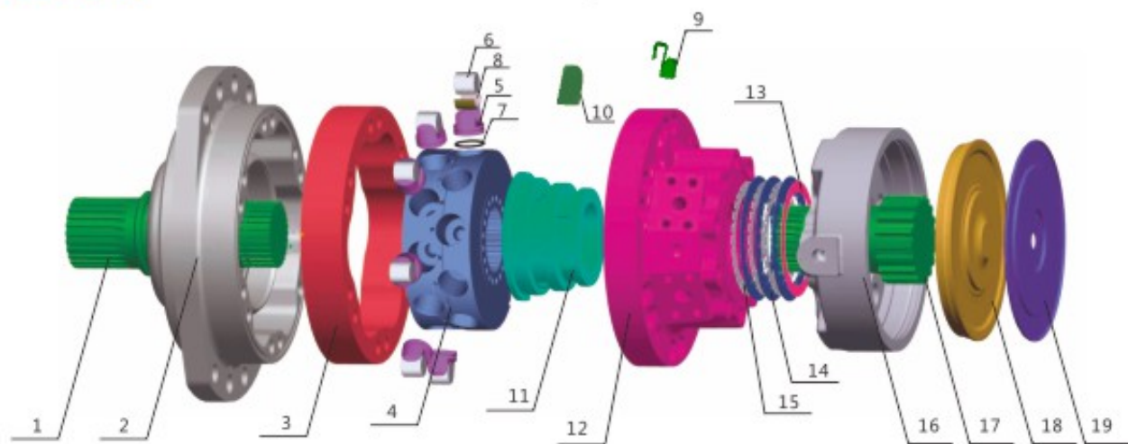
HMS50 系列零件名称表 HMS50 series parts list
